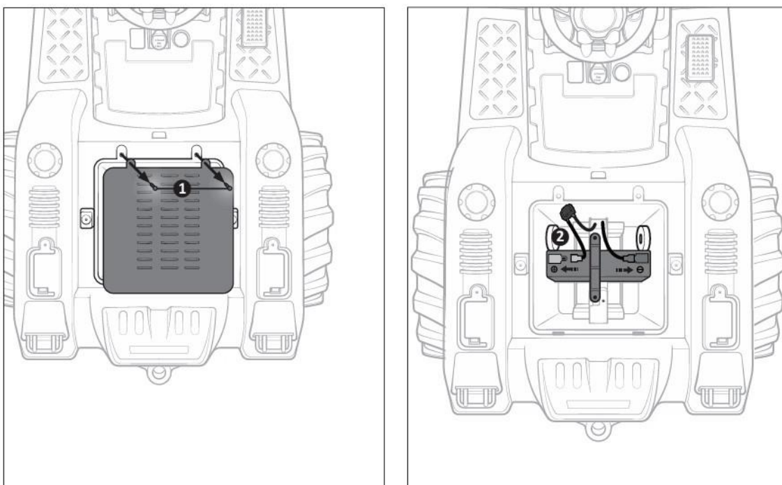
Obr. 1: Naskrutkujte plastový kryt. Obr. 2: Pripojenie batérie (pod sedadlom) - červený kábel na červený (+) kontakt batérie, čierny kábel na čierny (-) kontakt batérie.
